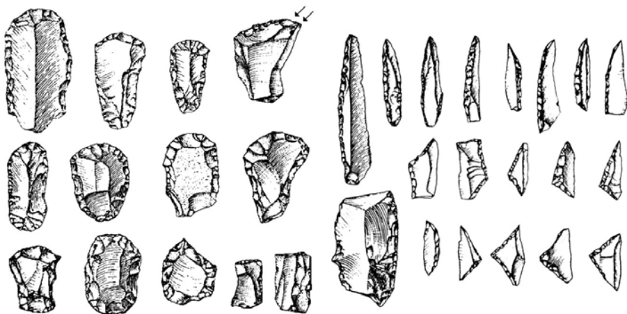
L'industria litica della Grotta di S. Teodoro (disegno da Vigliardi)
